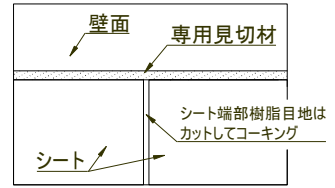
M-M' 断面
