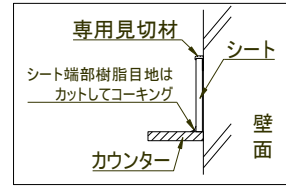
M-M' 断面
