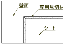
C部拡大
